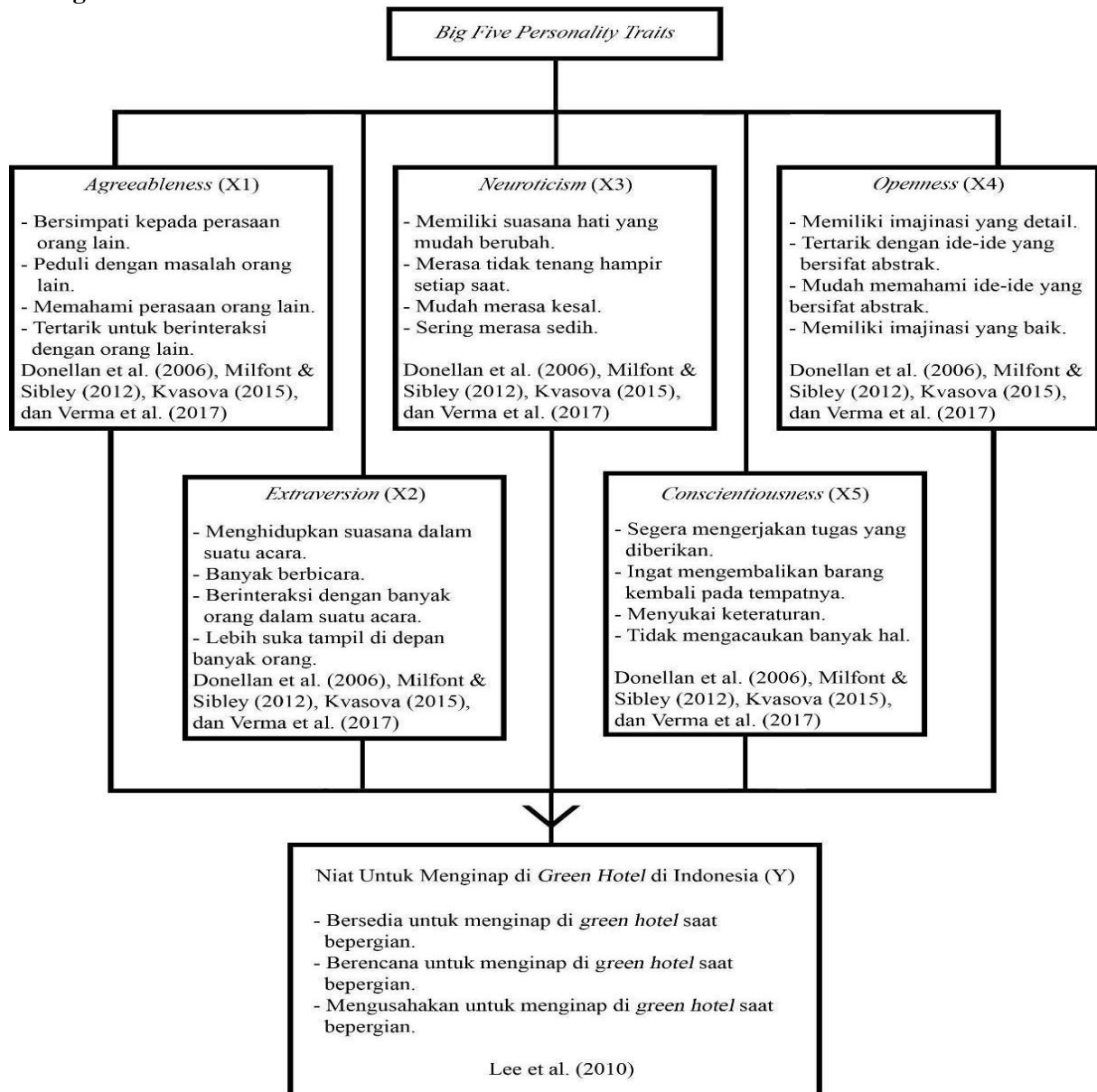
Gambar 1. Kerangka Pemikiran
